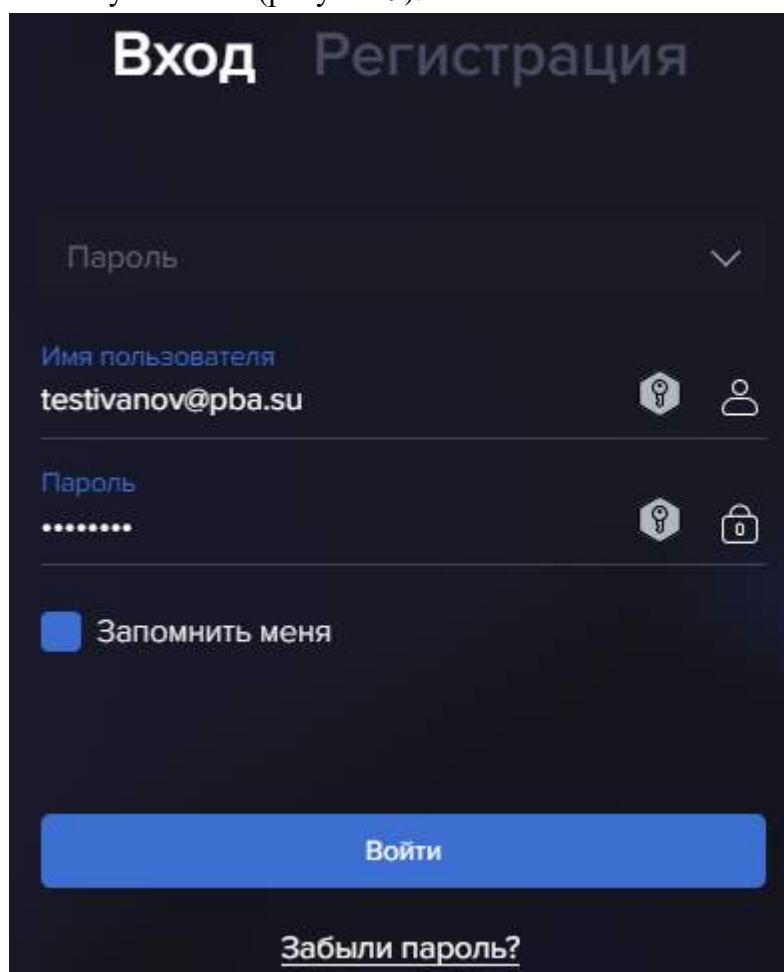
Рисунок 9 – Аутентификация
